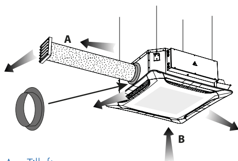
A = Tilluft B = Frånluft
